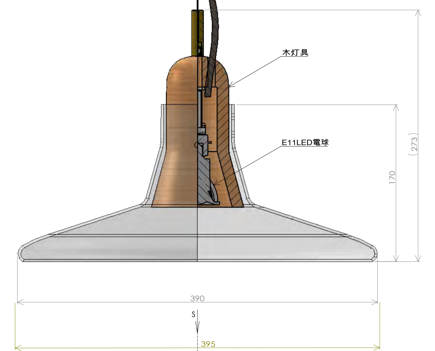
断面図 S-S
