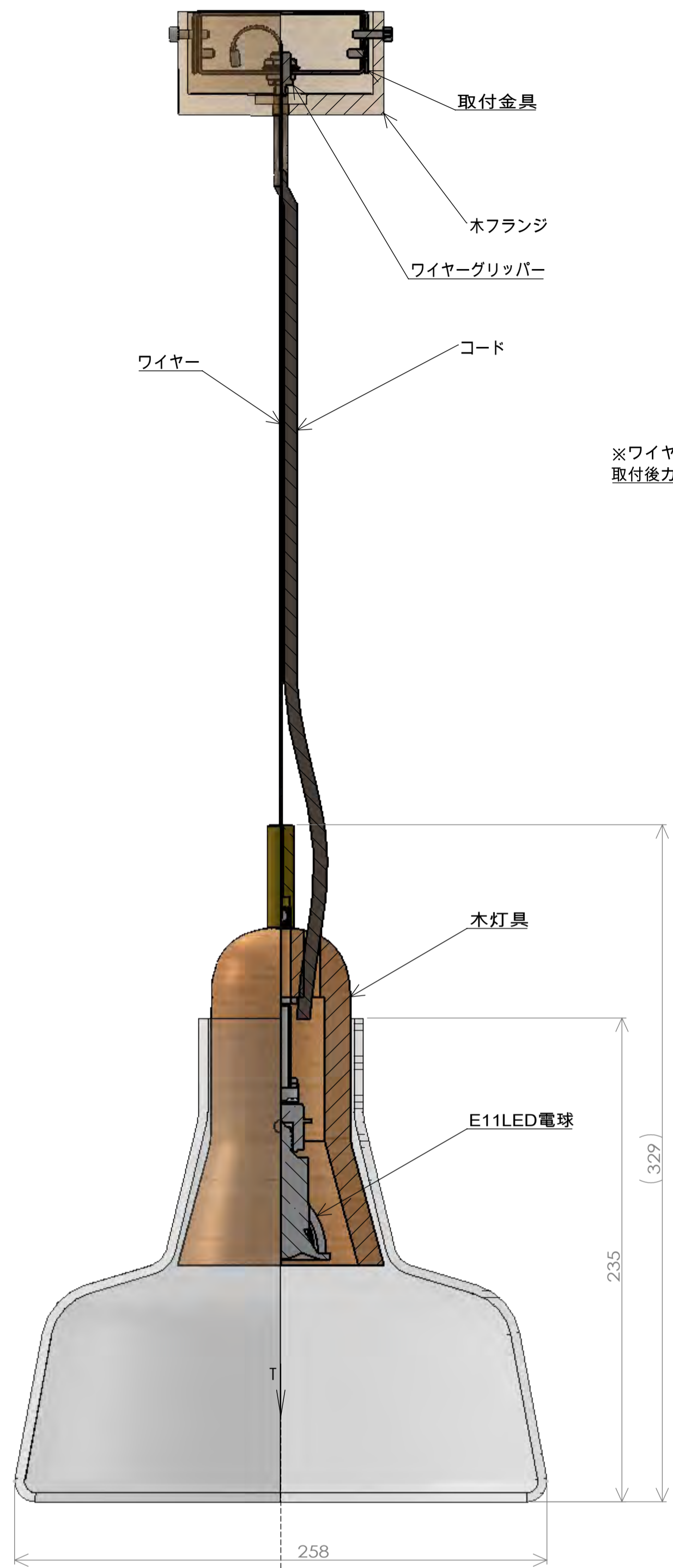
断面図 T-T
